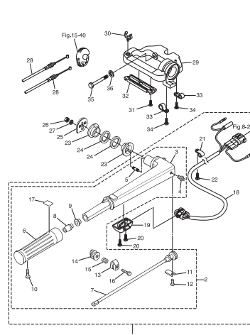
Fig. 14 TILLER HANDLE ティラハンドル
