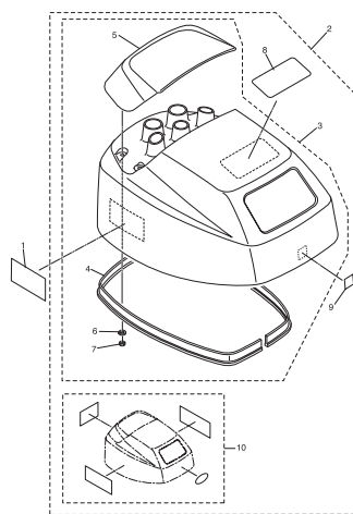
Fig. 18 TOP COWL トップカウル
